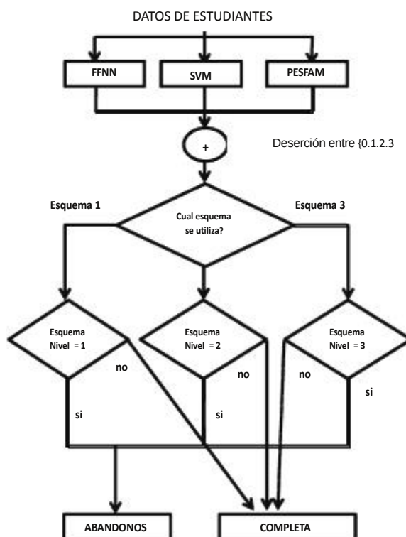
Figura 5. Esquema de decisión usada por el método propuesto
