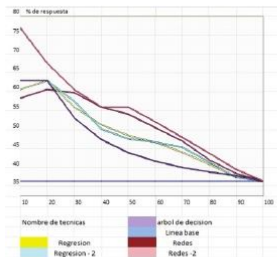
Figura 4. Evaluación y comparación de modelos
