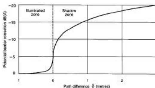
Figura 5. Corrección de la barrera potencial en función de la diferencia de trayectoria.
