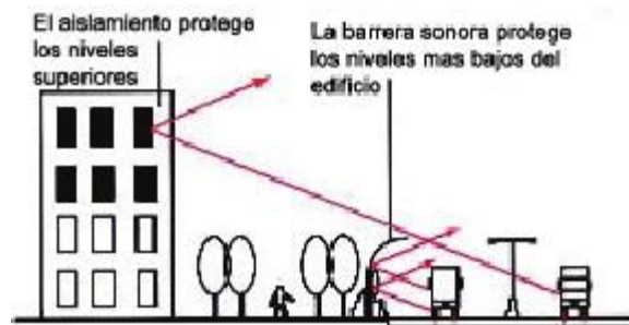
Figura 6. Forma de protección de una barrera voladiza.
