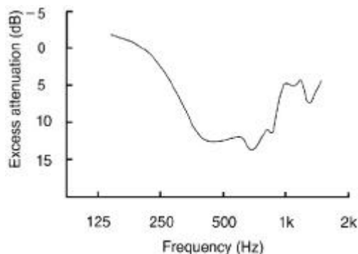
Figura 3. Atenuación excesiva por propagación sobre una base suave.
