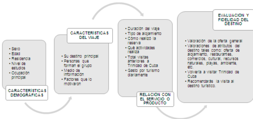
Diagrama 1 Listado de variables de segmentación
