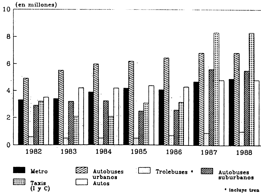
Figura 3a Distribución modal de pasajeros transportados (1982-1987) en el AMCM
