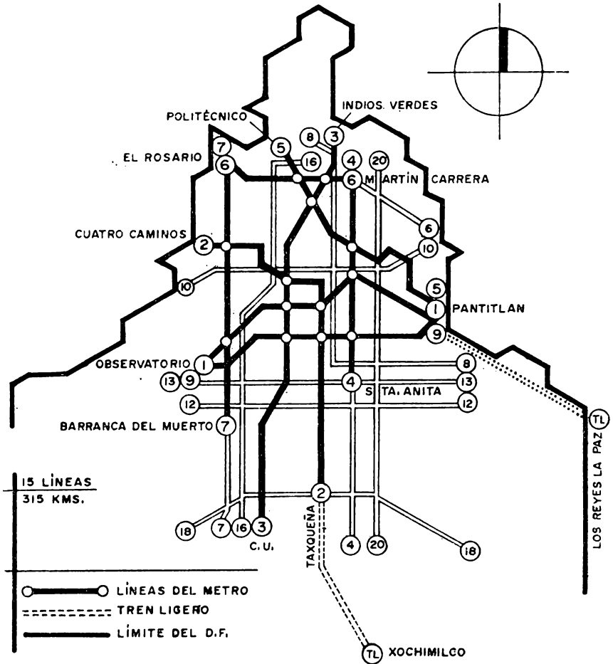
FIGURA 7 | PROYECCIÓN DE LA RED DEL METRO EN LA CIUDAD DE MÉXICO PARA EL AÑO 2010
