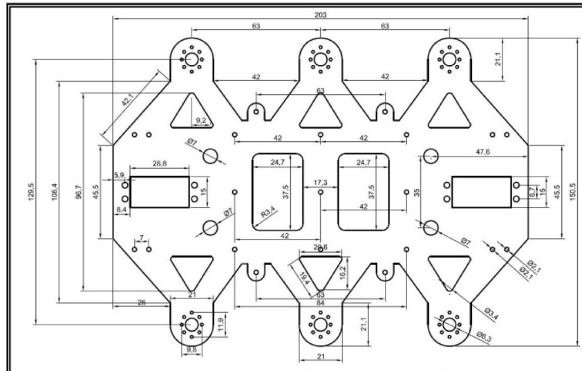
Figura 8. Plano del chasis del módulo hexápodo
