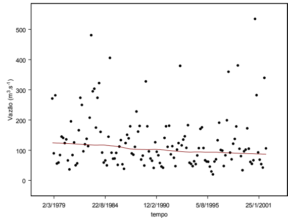
Figura 3 - Regressão RLWRS para o posto de vazão do rio Piracicaba 4D-007, (1979-2001).
