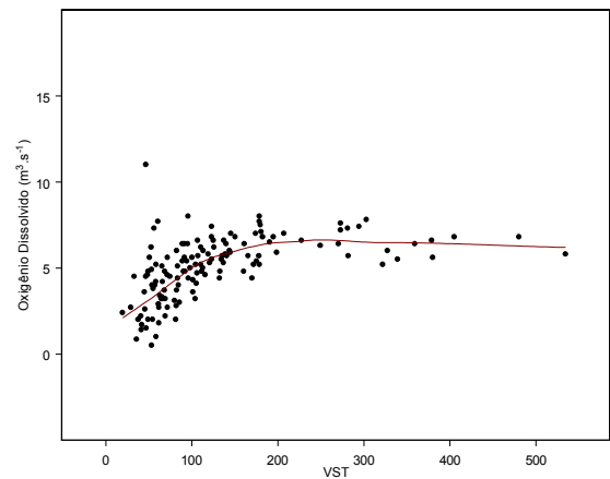
Figura 4 - Regressão RLWRS para OD, posto do rio Piracicaba (PI)
