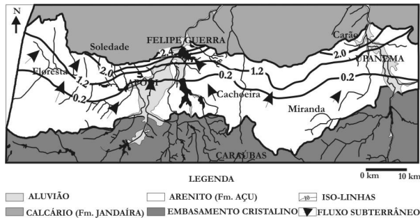
Figura 6 - Iso-valores de condutividade hidráulica (m/d) do aquífero Açú
