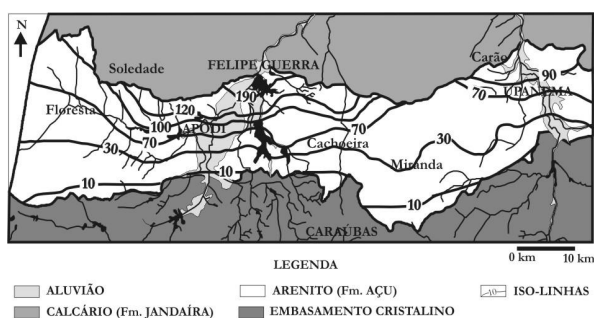
Figura 4 – Iso-valores de espessura saturada (m) do aquífero Açú
