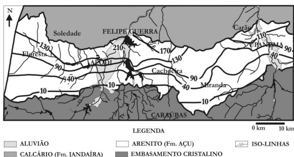
Figura 3 – Iso-espessura (m) da Formação Açú
