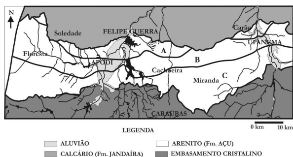
Figura 11 – Avaliação potencial do aquífero Açú
