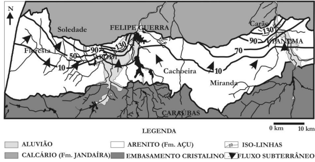
Figura 5 – Iso-valores de transmissividade (m 2 /d) do aquífero Açú
