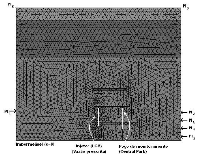
Figura 3 - Malha bidimensional vertical de elementos finitos utilizada nas simulações numéricas.
