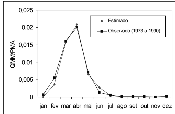
Figura 3 – Escoamento superficial mensal, médio ponderado, observado e estimado pelo modelo, em escala diária, para a bacia hidrográfica do açude Epitácio Pessoa
