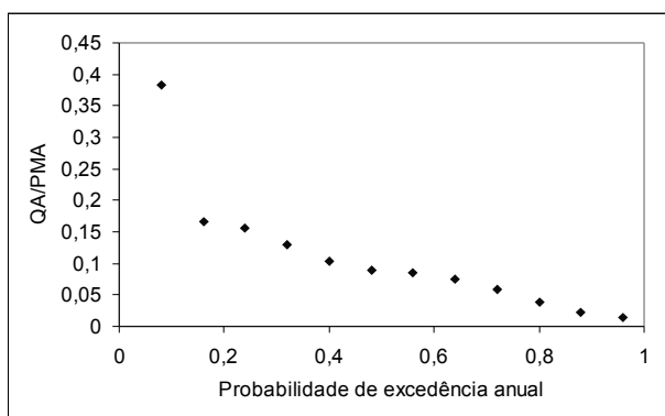
Figura 13 – Estimativa do escoamento superficial anual estimado pelo modelo para a bacia hidrográfica do açude Epitácio Pessoa
