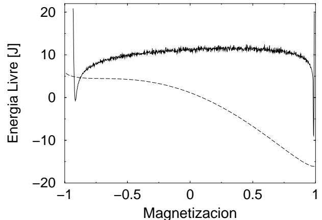
Figura 12. Comparación de la energía libre como función de la magnetización. Línea continua simulación y línea punteada campo medio.
