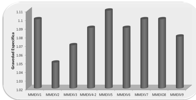
Figura 1. Gravedad específica en genotipos de yuca
