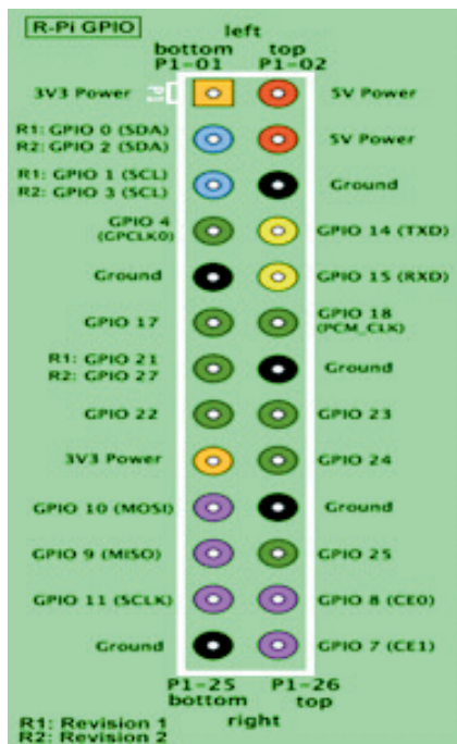
Figura 2. Asignación de pines GPIO en la Raspberry Pi Modelo B, rev 1 y Modelo B, rev 2 (General Purpose Input/Output (GPIO), 2015)
