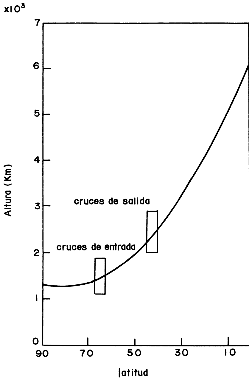
Fig. 17. Comparación de la altura de la ionopausa nocturna observada, con la predicción del modelo de entrada polar. (Pérez de Tejada, 1980).
