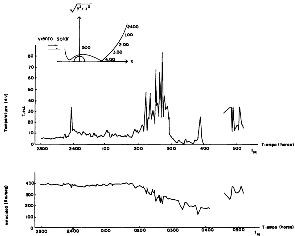
Fig. 11. Comportamiento de la velocidad y temperatura del plasma según observaciones realizadas en la estela del planeta con el vehículo Venera 9 (Romanov et al. , 1979).
