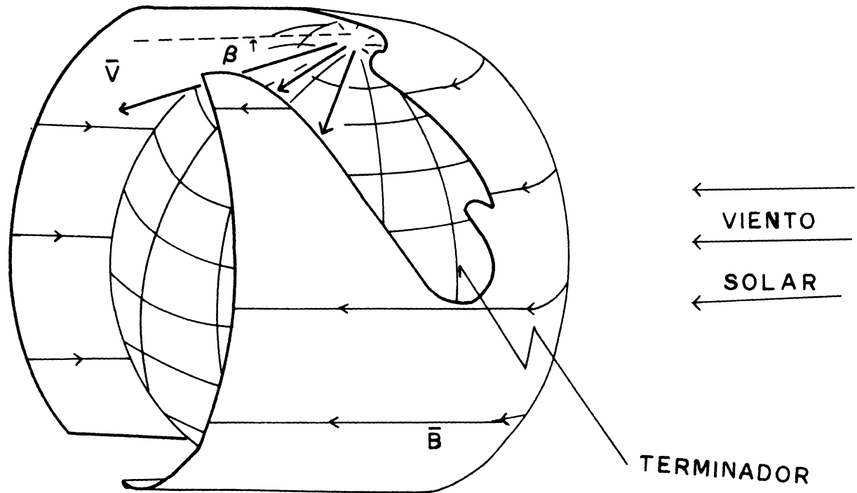
Fig. 16. Diagrama de la entrada del viento solar por las regiones polares del terminador planetario. (Pérez de Tejada, 1980).
