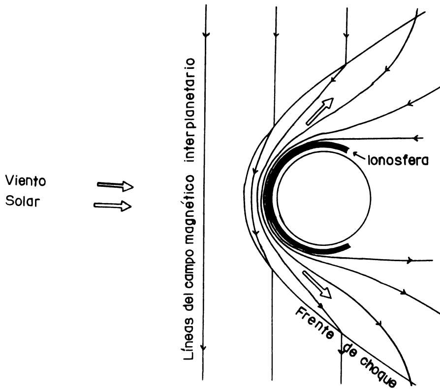
Fig. 5. Diagrama de la deformación y acumulación de las líneas del campo magnético interplanetario alrededor del obstáculo ionosférico. Las líneas de campo descansan usualmente sobre el plano de la eclíptica y pueden suponerse perpendiculares a la dirección de movimiento del viento solar. (Johnson y Hanson, 1979).
