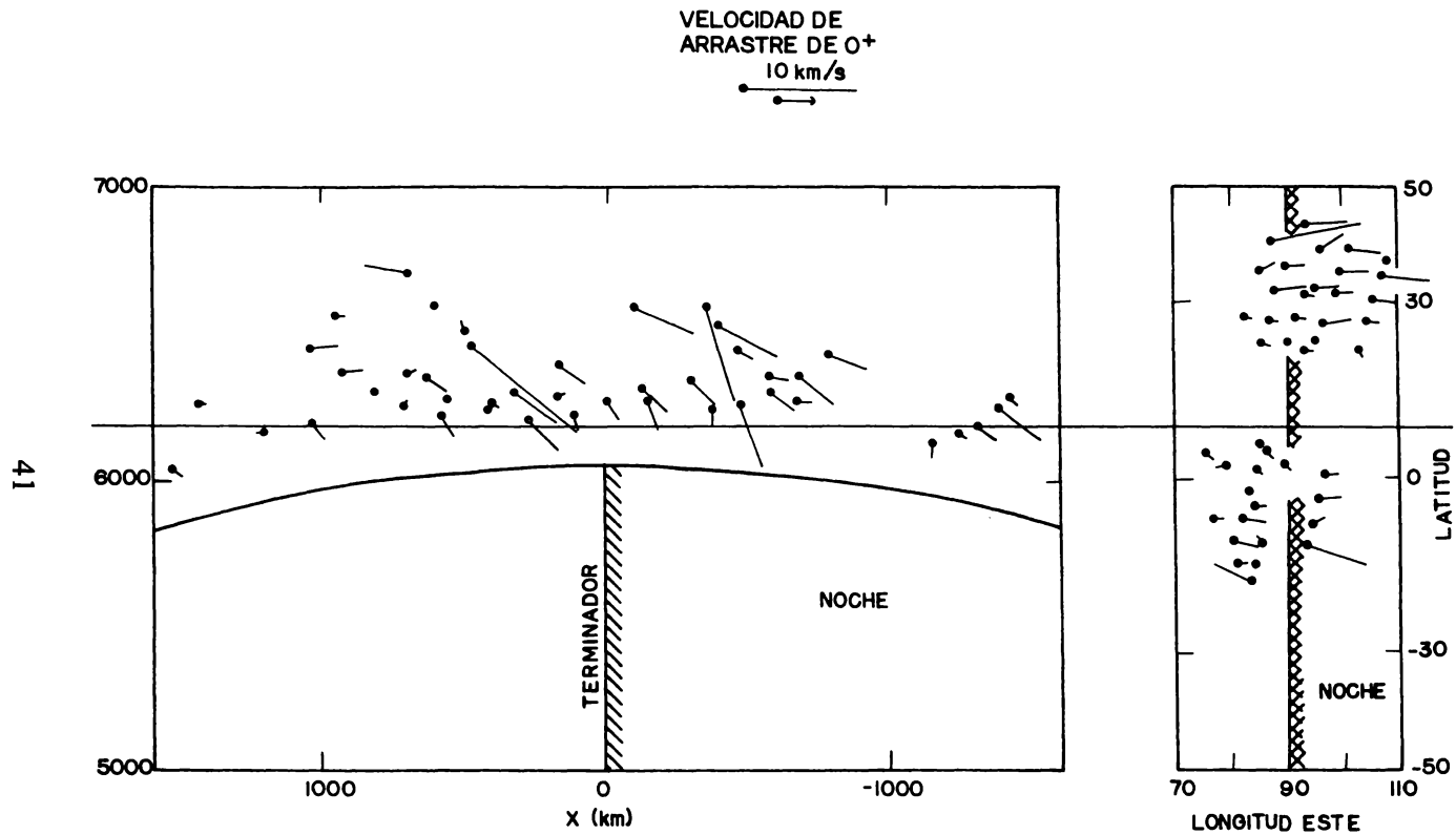
Fig. 13. Dirección de movimiento de partículas ionosféricas cerca del terminador según observaciones realizadas con el Pionero Venus. Los vectores velocidad están trazados a partir de las posiciones de medición. (Knudsen et al. , 1980).
