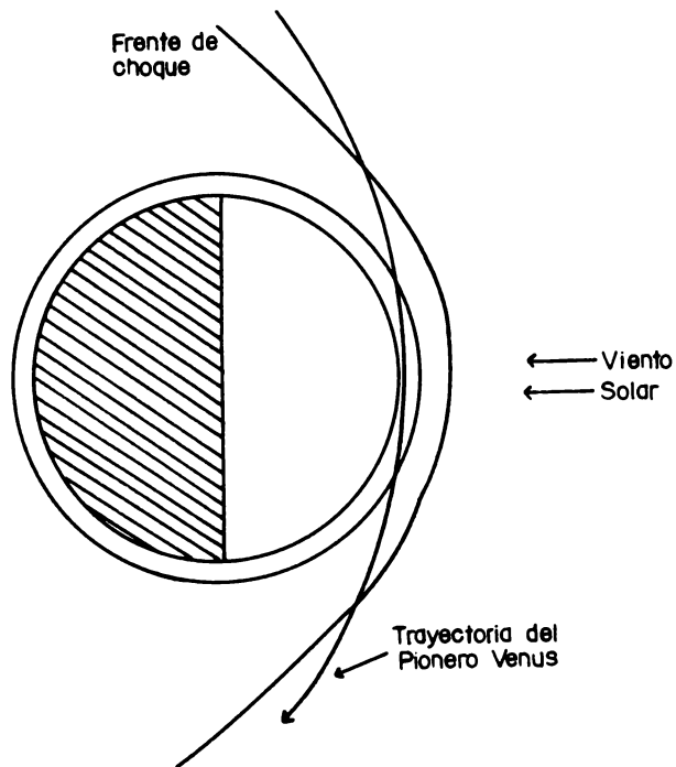
Fig. 6. Registro magnético a lo largo de la Trayectoria del Pionero Venus. Las discontinuidades observadas para t < -26 min y t > 40 min corresponden al cruce del satélite por el frente de choque. Movimientos repentinos de éste, debidos a cambios en la velocidad del viento solar, pueden dar lugar a cruces múltiples como ocurrió para t > 40 min en la órbita mostrada. El diagrama inferior muestra la trayectoria proyectada sobre el plano perpendicular al de la eclíptica. (Russell et al. , 1979).
