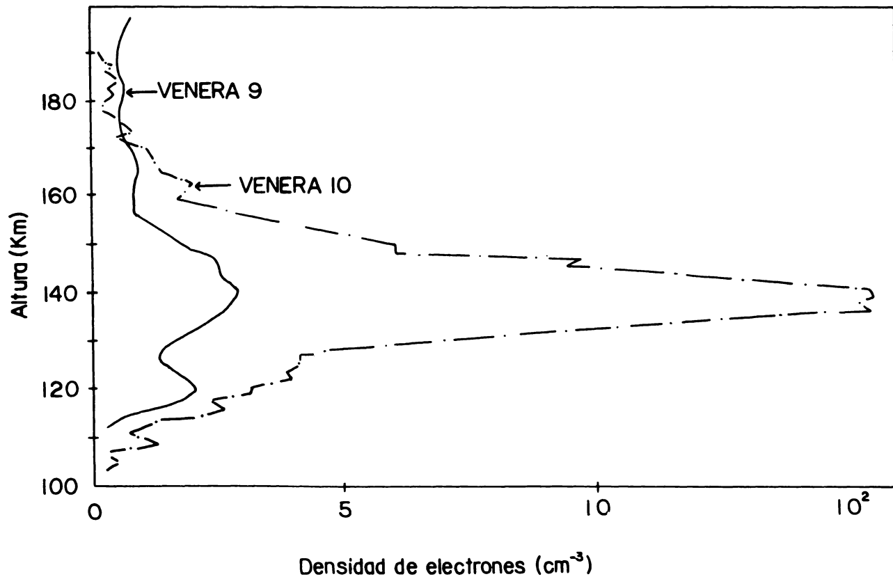
Fig. 18. Perfil ionosférico sobre el hemisferio noche. (Breus, 1979).
