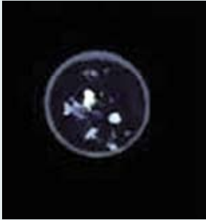
Figura 22. Reacciones positiva y negativa de cepas expuestas a reactivos de superoxol (H 2 O 2 al 30%) y de catalasa (H 2 O 2 al 3%).
