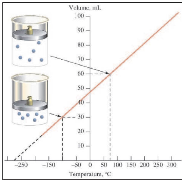
Figura 2. Ley de Charles.
