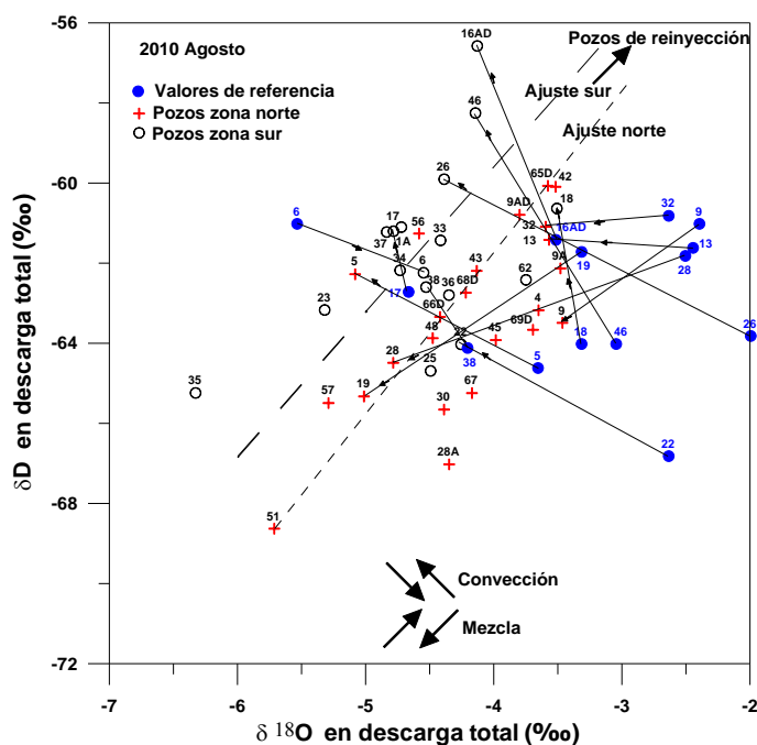
Fig. 9. Composición isotópica de agosto de 2010 de fluidos de pozos de Los Azufres y valores de referencia.
