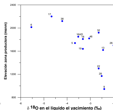
Fig. 4. Concentración de O-18 en la fase líquida del yacimiento según datos de referencia dados en el modelo geoquímico conceptual vs elevación de las zonas productoras de los pozos (Nieva et al., 1987).
