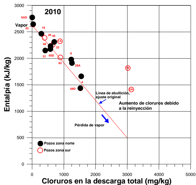
Fig. 8. Comportamiento entalpía vs cloruros de pozos de mezcla según datos de 2010.
