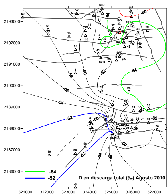
Fig. 10. Distribución de valores de \delta D en la descarga total de pozos productores según datos de agosto de 2010.
