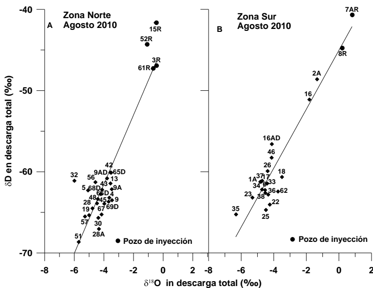
Fig. 7. δD vs δ 18 O de fluidos de pozos del campo geotérmico de Los Azufres según datos de 2010.
