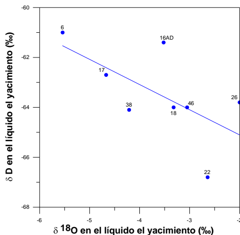
Fig. 5. Oxígeno-18 vs deuterio en la fase líquida del yacimiento de pozos de la zona sur, según datos de referencia dados en el modelo geoquímico conceptual (Nieva et al., 1987).
