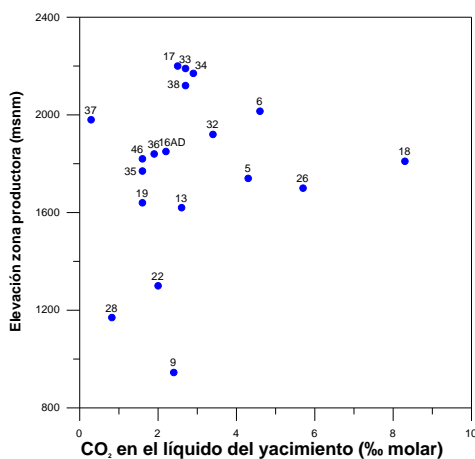
Fig. 2. Concentración de \text{CO}_2 en la fase líquida del yacimiento según datos de referencia dados en el modelo geoquímico conceptual vs elevación de las zonas productoras de los pozos (Nieva et al., 1987).
