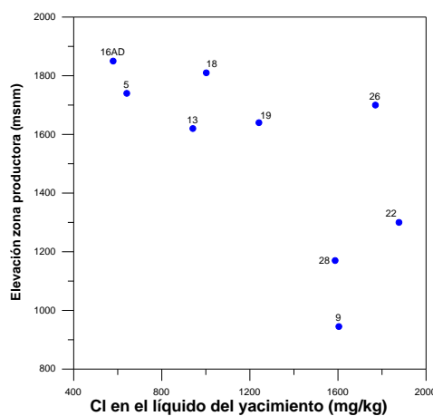
Fig. 3. Concentración de Cl en la fase líquida del yacimiento según datos de referencia dados en el modelo geoquímico conceptual vs elevación de las zonas productoras de los pozos (Nieva et al., 1987).
