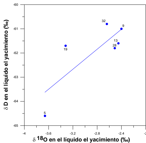
Fig. 6. Oxígeno-18 vs deuterio en la fase líquida del yacimiento de pozos de la zona norte, según datos de referencia dados en el modelo geoquímico conceptual (Nieva et al., 1987).
