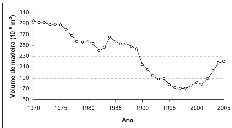
Figura 2 – Evolução do consumo de madeira para energia no Brasil – 1970 a 2005 (Ministério..., 2007a).
