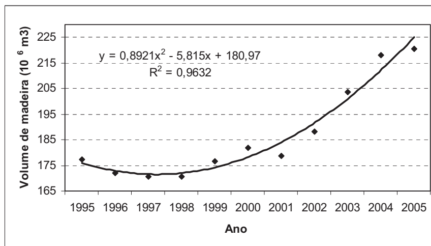
Figura 3 – Evolução do consumo de madeira para energia no Brasil – 1995 a 2005 (Ministério..., 2007a).
