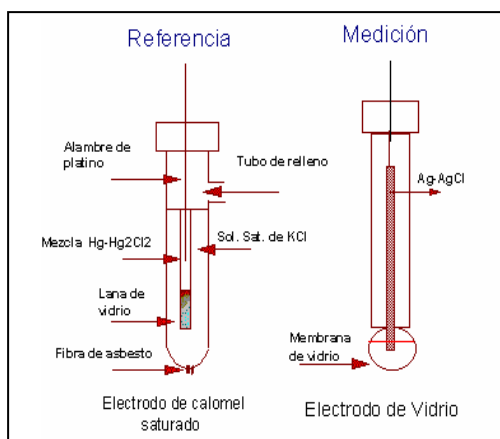
Figura 1. Electrodos utilizados en la medición del pH.
