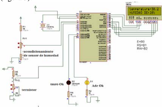
Figura 5. Sistema trabajando en su conjunto.
