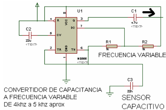
Figura 2. Convertidor de capacitancia a frecuencia.
