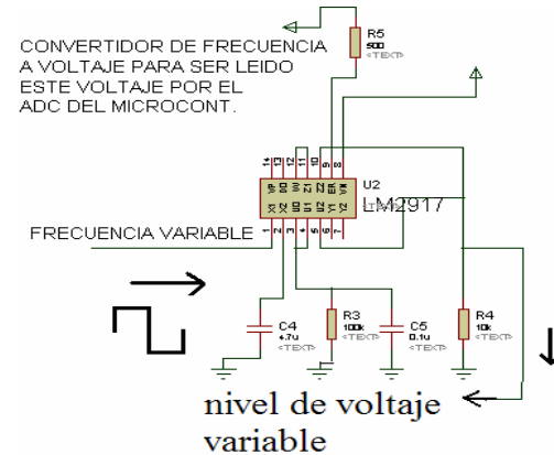
Figura 3. Convertidor de frecuencia a voltaje.
