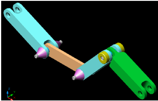
Fig. 2. Segunda propuesta para la cadena cinemática del banco experimental.
