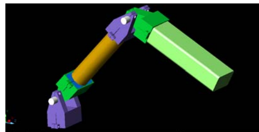
Fig. 8.- Tercera Propuesta aquí se resuelve el problema para articular con pasador formando una sencilla revoluta. Los eslabones de diferentes medidas en longitud y geometría, podrán intercambiarse en la posición de la cadena de n eslabones.
