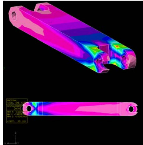
Fig. 10.- Se puede observar como la concentración de esfuerzos queda aislada en zona cercana a la articulación básicamente en el contacto con el perno y que entonces una extensa zona central del elemento presenta mejor grado de homogeneidad para el estudio de los esfuerzos debidos a flexión pura.
