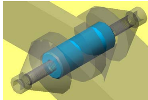
Fig. 4.- Se muestra el eje de revoluta dentro del ensamble de articulación y los eslabones
