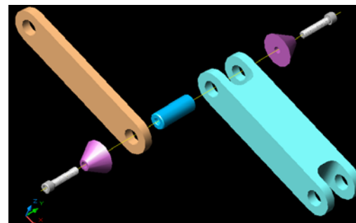
Fig. 7.- Sub-ensamble de segundo modelo propuesto
