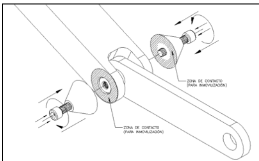
Fig. 6.- Manera de inmovilizar las articulaciones de revoluta: El apriete de los tornillos empuja las roldanas contra las paredes exteriores, impidiendo el deslizamiento entre tales superficies.
