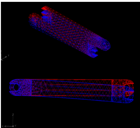
Fig. 9.- Vista oblicua y lateral del eslabón, donde la forma del elemento descargado, y el elemento cargado puede simularse
