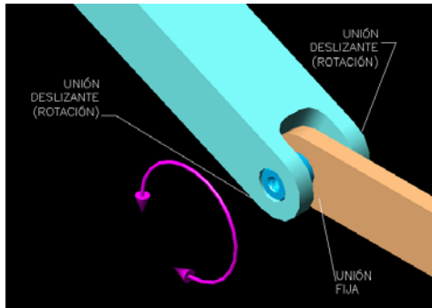
Fig. 5.- Detalle de sub-ensamble de eslabón de doble herradura (azul), eslabón simple (café claro) y flecha. La flecha color púrpura indica la dirección de movimiento o rotación relativo entre los eslabones.
