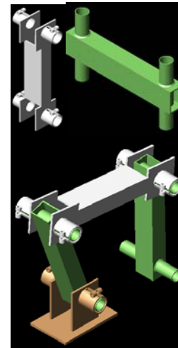
Fig. 1.- Primera propuesta para la cadena cinemática del banco experimental.
