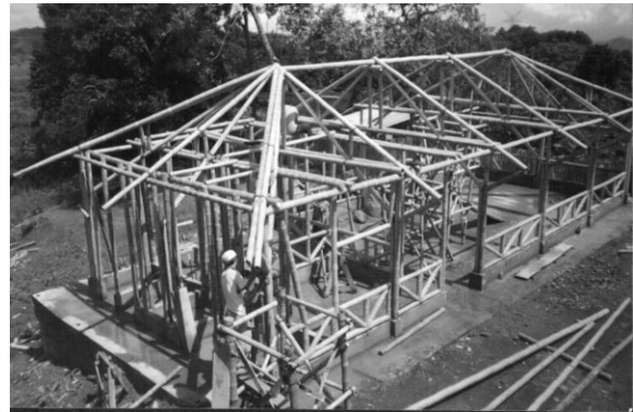
Foto 1.- Casa Habitación (desplante de columnas y vigas de Bambú) 1
