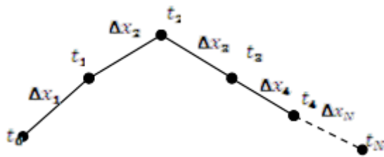
Figura 2.: Trayectoria recorrida por un electrón desde x_0 hasta x_N . En resumen, la expresión (11) se puede escribir
