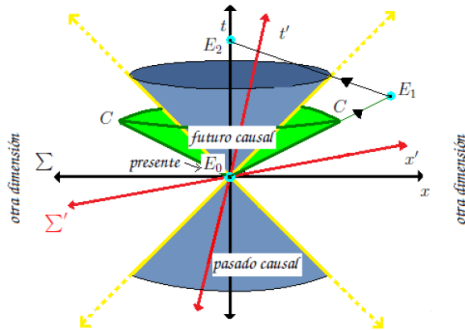
FIGURA 1: (a) Paradoja al usar taquiones. E_0 , E_1 , y E_2 corresponden a eventos que están casualmente conectados y dependen del envío de taquines. (b) Propagación del taquion sin paradojas casuales. Ambas señales viajan a futuro en un sistema de referencia en reposo \Sigma .
