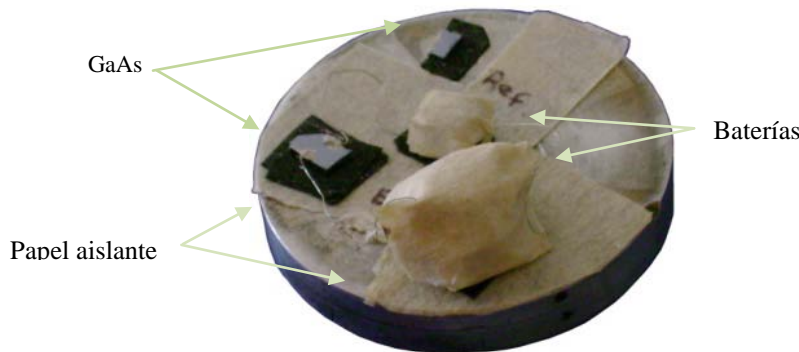
Figura 1: Montaje experimental.
