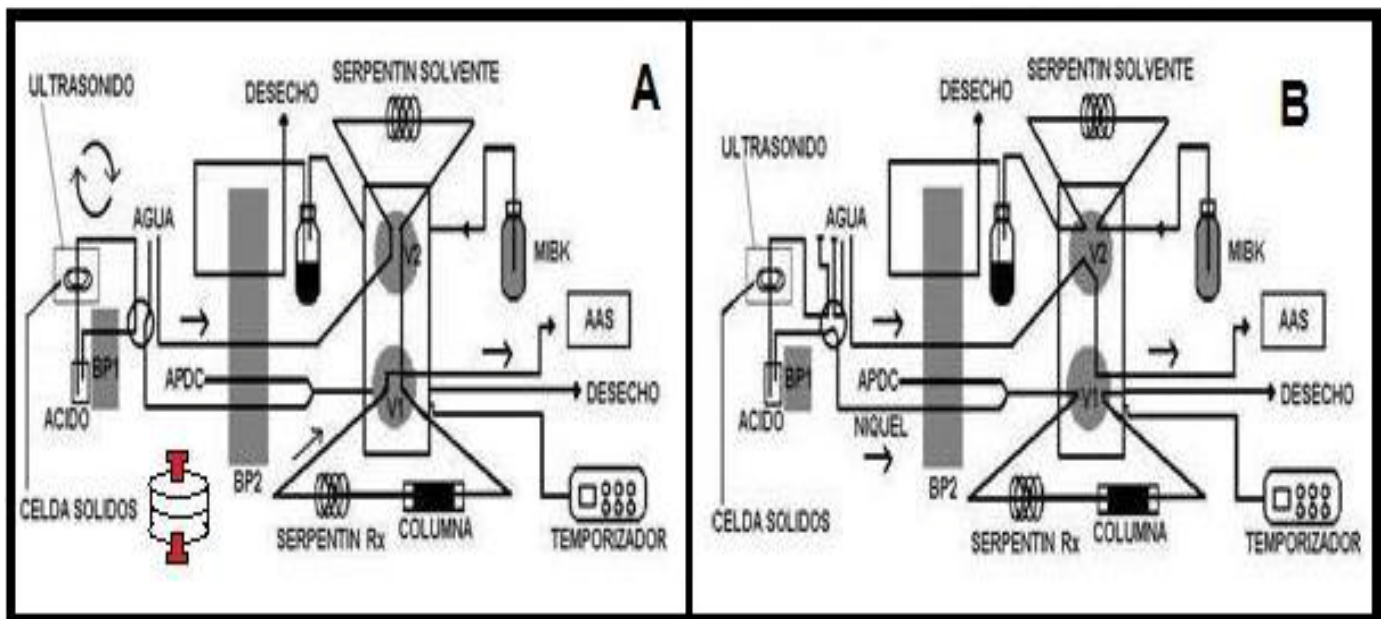
Figura 1: Configuración de flujo empleada. A: Etapa de extracción-elución. B: Etapa de Inyección-preconcentración. Todos los caudales óptimos se indican en la Tabla 1.
