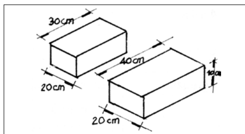
Figura 12: Medidas típicas de adobes en la zona andina.
