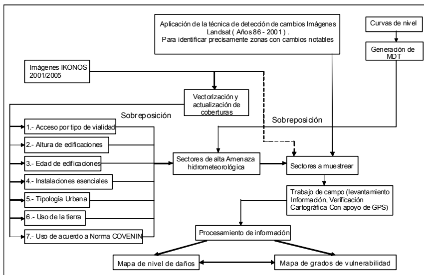
Figura 2. Esquema metodológico para la extracción de información temática con el uso de datos de sensores remotos
