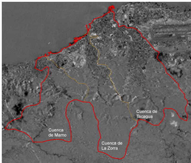
Figura 14. Imagen resultante. Producto de la substracción (Marzo 86-Marzo 01)
