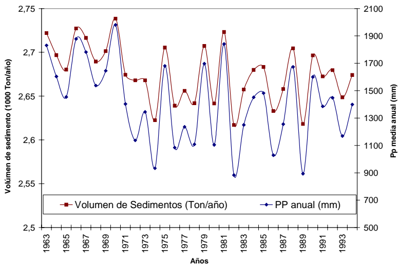
Figura 3. Valores estimados de los volúmenes de sedimentos y la pp anual en la cuenca de la quebrada San Ignacio. Período (1963-1994). Laguna de Tacarigua, estado Miranda
