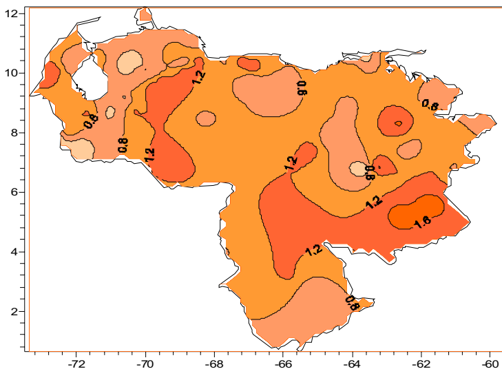
Figura 9. Precipitación media diaria (mm) y probabilidad de ocurrencia de precipitación (%). Procesos extremos bimestre julio-agosto (1956-1977).
