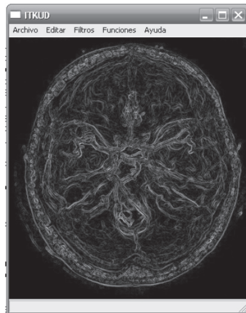
Figura 9. Gradiente.
