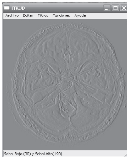
Figura 18. Operador Sobel.
