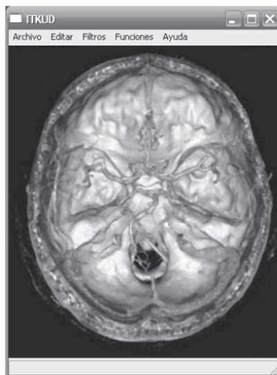
Figura 13. Mediana.
