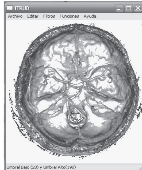
Figura 5. Umbralización.
