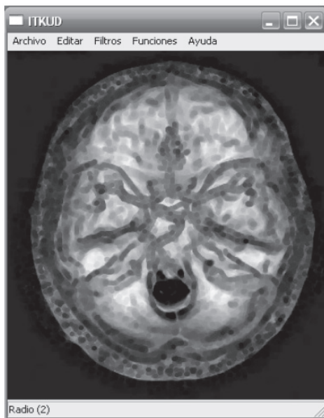
Figura 10. Erosión.
