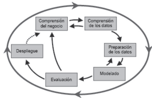
Figura 6. Ciclo CRISP.
