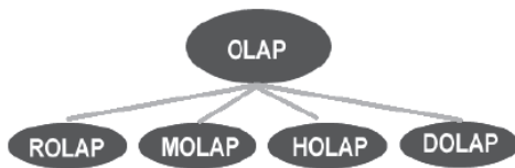
Figura 1. Subdivisión OLAP.
