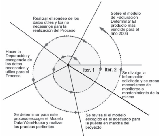
Figura 7. Proceso CRISP.
