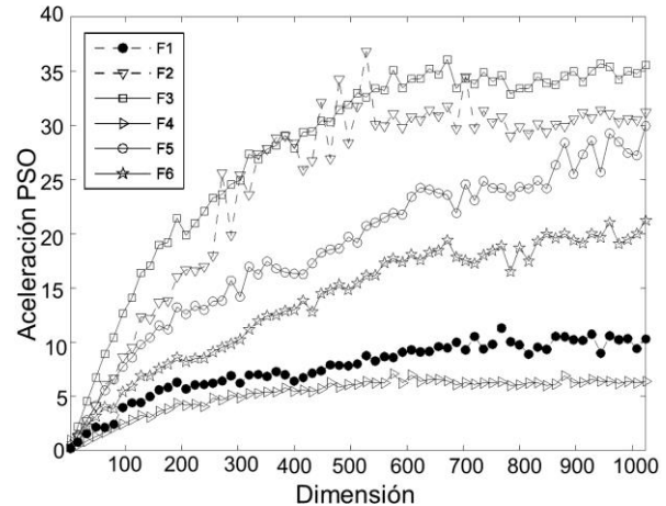
Fig. 2. Aceleración vs. dimensiones en el algoritmo PSO. Fuente: Autores
