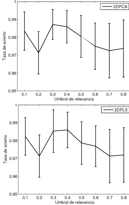
Fig. 5. Sintonización del umbral de relevancia
