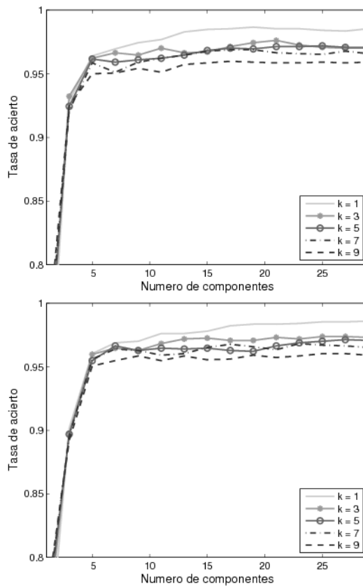
Fig. 6. Sintonización del número de vecinos del clasificador y el número de componentes en los métodos de descomposición lineal
