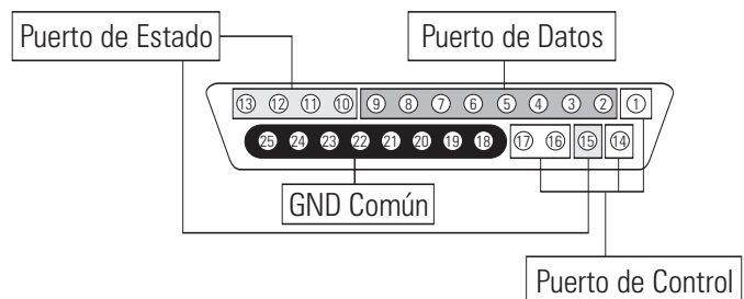
Fig. 2 Estructura física del puerto paralelo
