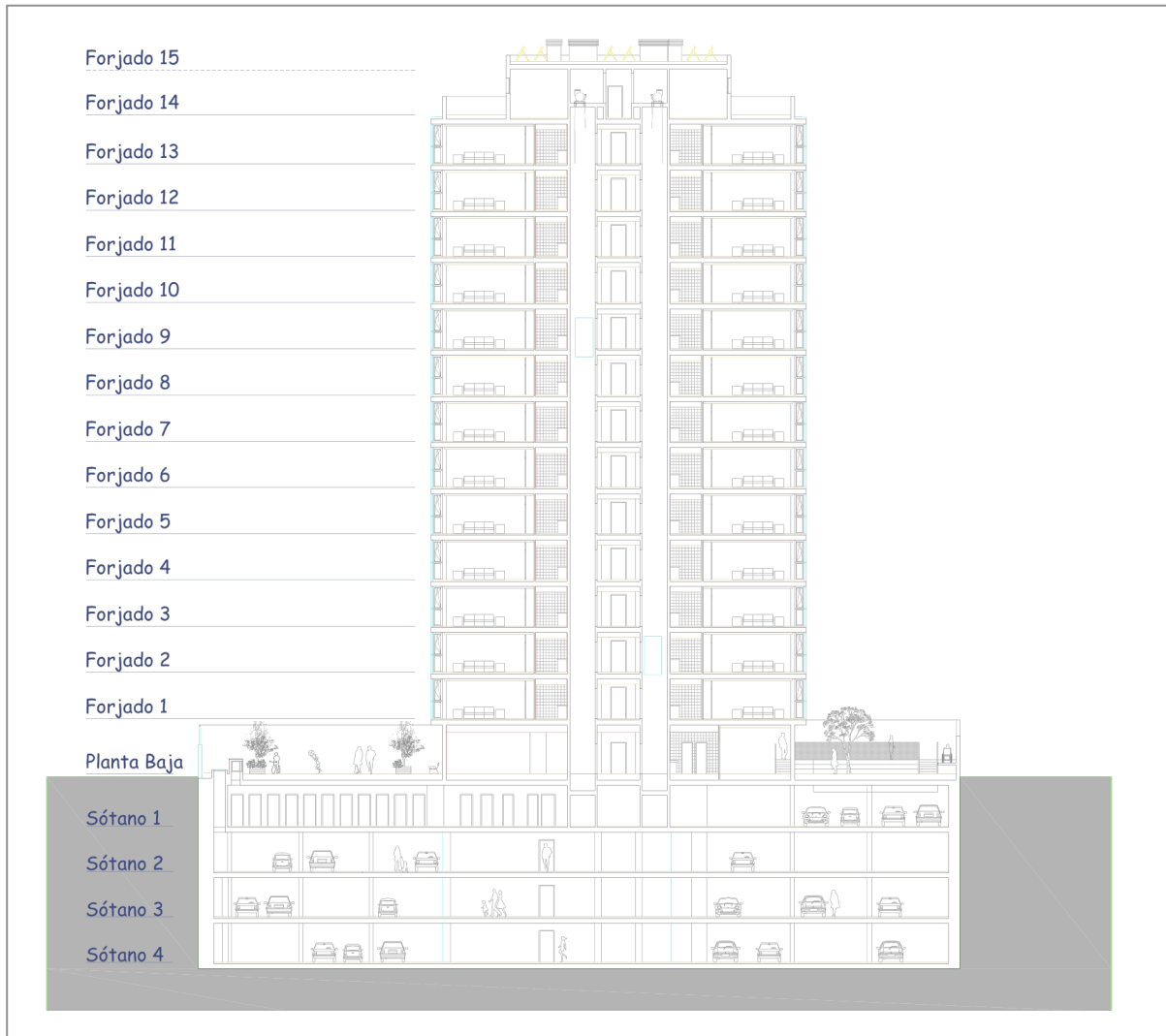
Figura 1. Sección del edificio
