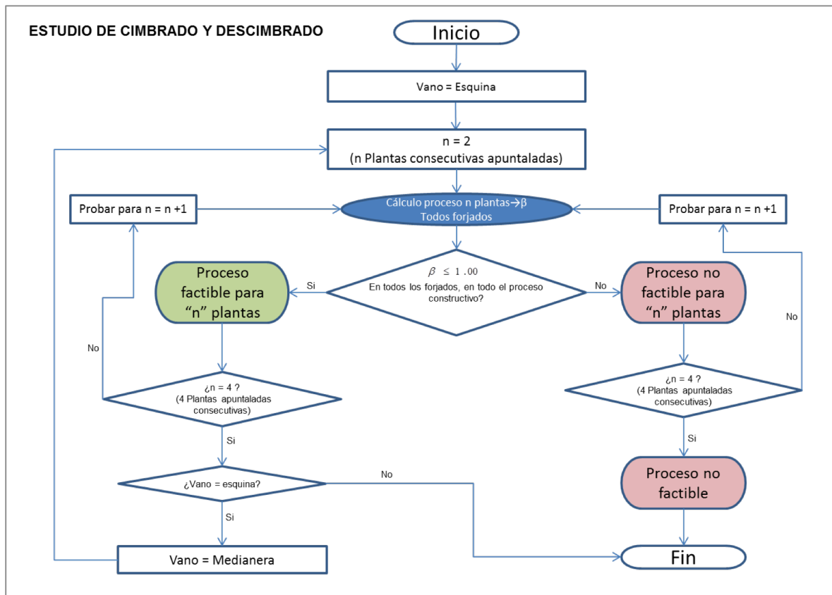
Figura 3. Procedimiento de análisis de proceso de cimbrado y descimbrado factibles para el edificio objeto de este estudio
