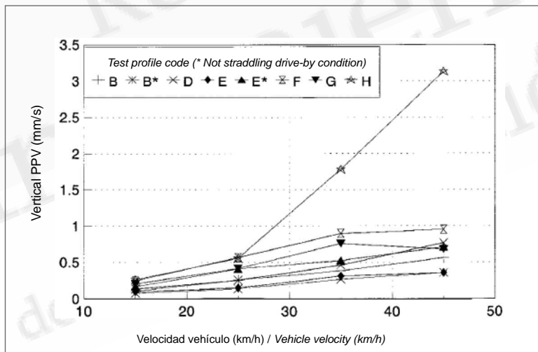
Figura 1. Velocidad PPV (ordenadas) contra Velocidad del vehículo articulado km/h (abscisas). (G.R. Watts a, 2000) Figure 1. PPV Velocity (ordinates) against articulated vehicle Velocity km/hr (abscises). (G.R. Watts a, 2000)
