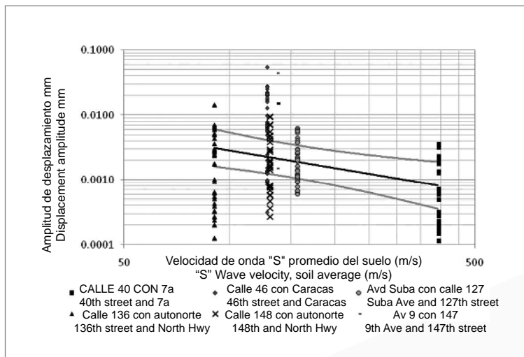
Figura 16. Correlación de la amplitud de desplazamiento de los lugares instrumentados en función de la velocidad de onda de los lugares bajo estudio
