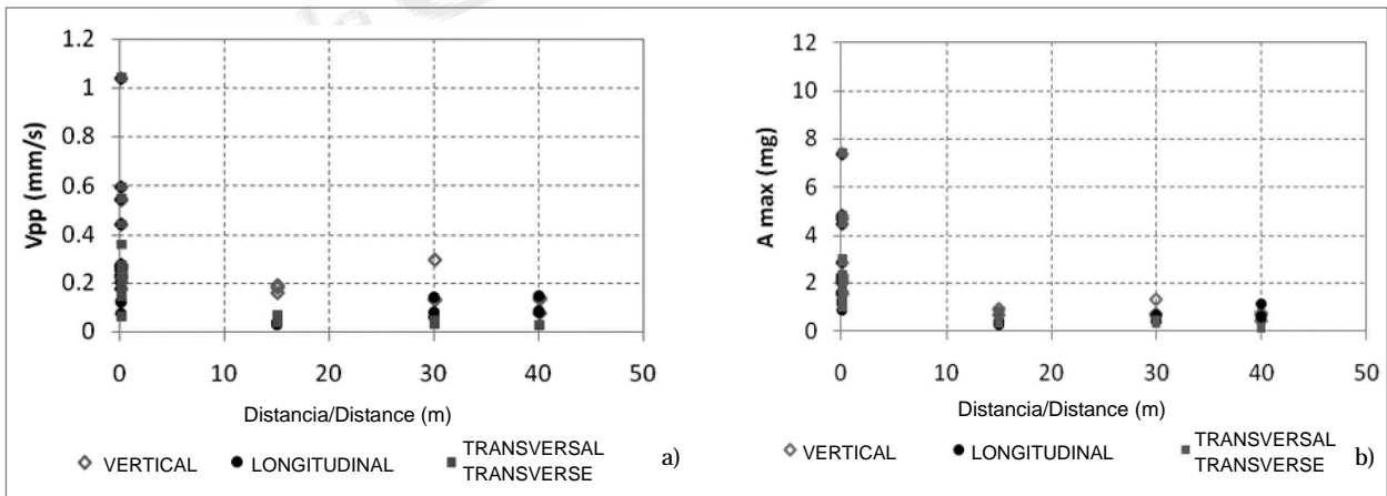
Figura 11. Atenuación de la aceleración (a) y de la velocidad (b) en los registros tomados en la Calle 136 con Autopista Norte Figure 11. Acceleration (a) and Velocity (b) attenuation in recordings measured at 136th Street and North Highway
