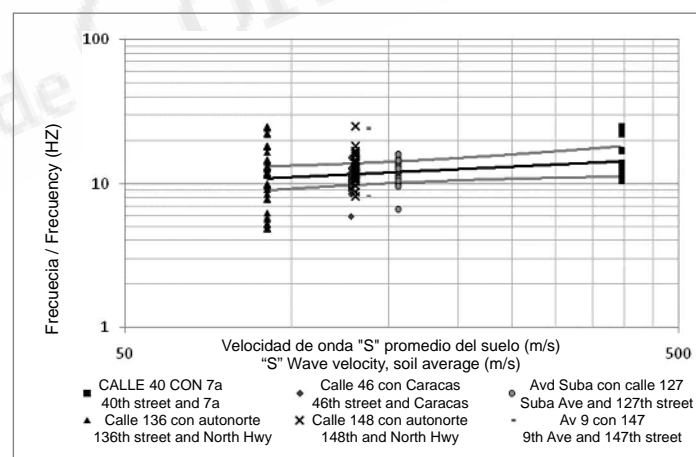
Figura 15. Correlación de la frecuencia de los registros en función de la velocidad de onda de los lugares bajo estudio
