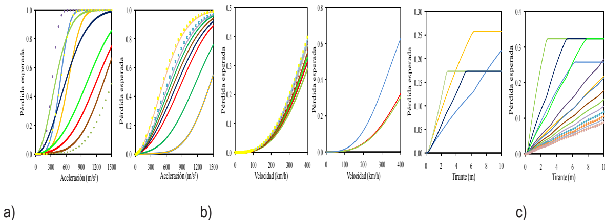
Figura 6. Funciones de vulnerabilidad para el sector salud: a) Sismo, b) Viento y c) Inundación
