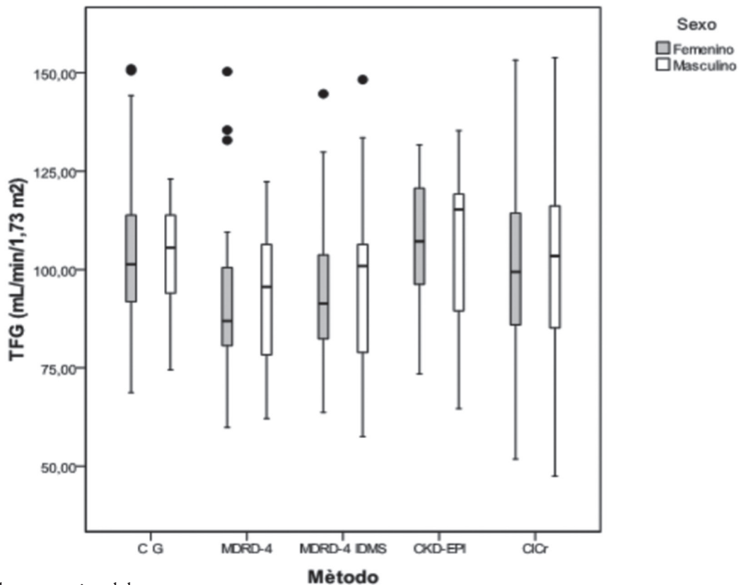
Figura 1. Diagrama de cajas y bigotes por método de estimación de TFG y por sexo
