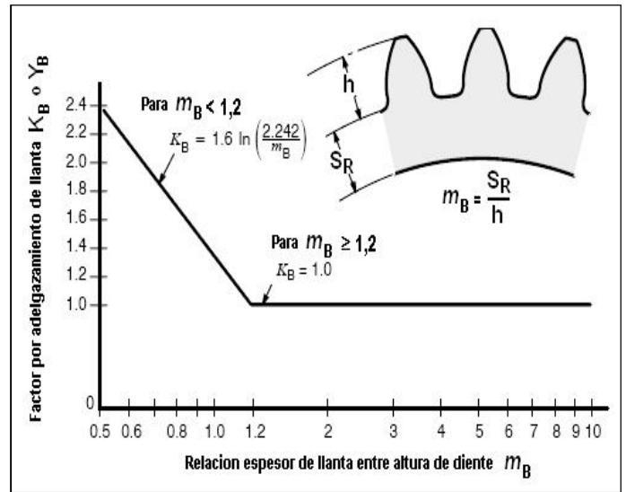
Fig. 6. Factor por adelgazamiento de llanta, K_B o Y_B [6, 7]
