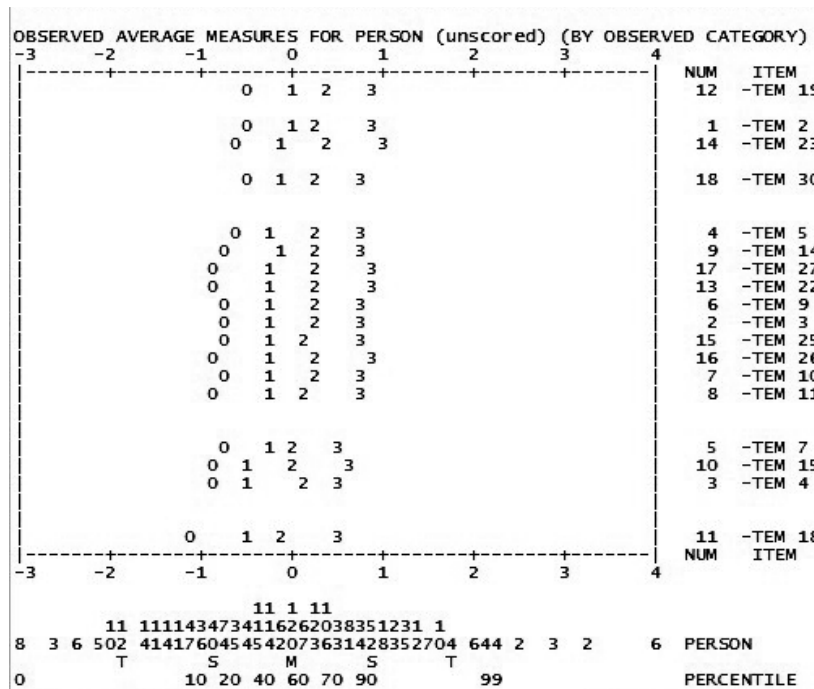
Figura 1. Mapa de las categorías de respuestas en los 18 ítems del cad-fs.
