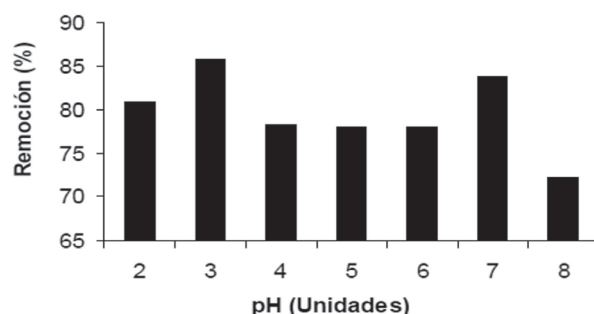
Figura 1. Influencia del pH en la remoción de Cr(VI) por cáscara de coco seca. Condiciones experimentales: C_0 = 1.84 \text{ mg/dm}^3 ; a = (2,91 \text{ s}^{-1}) ; C \text{ (biomasa)} = 5 \text{ g/dm}^3 y tiempo de contacto de 1 hora.
