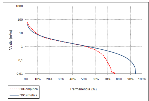
Figura 6 – Comparação entre as FDC's sintética e empírica na estação de Sítio Lapinha – \tau modelado
