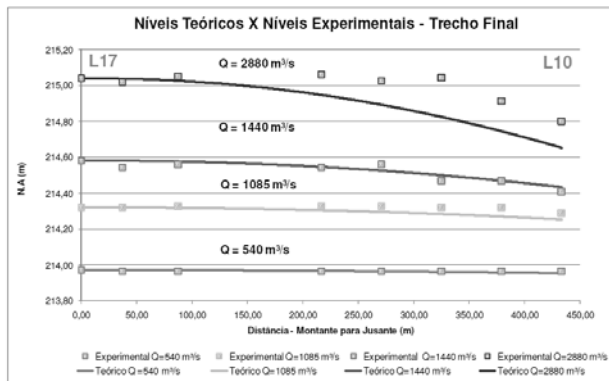
Figura 10 – Comparação dos níveis de água ao longo do canal para diferentes vazões
