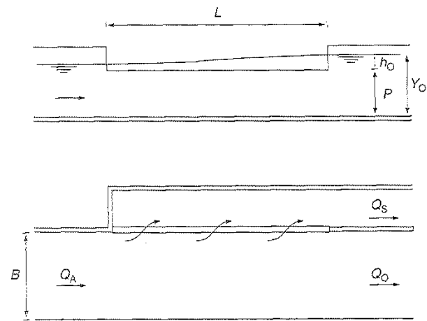
Figura 2 – Vertedouro lateral e canal lateral sob escoamento subcrítico (May et al., 2003)
