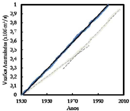
Figura 3 – Vazões Acumuladas Corrigidas para Salto Osório
