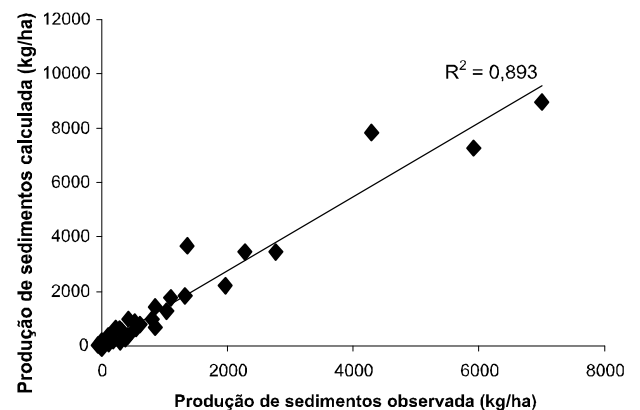
Figura 3 – Comparação da E_o com a E_c na M1BESJC com os parâmetros médios regionais
