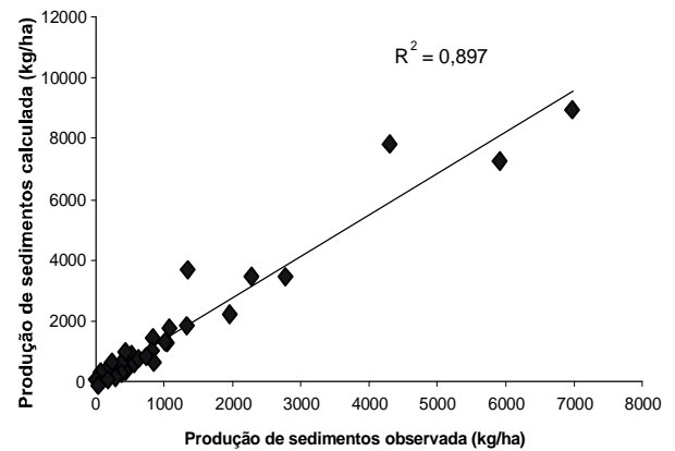
Figura 2 – Comparação da E_o com a E_c na M4BES com os parâmetros médios regionais
