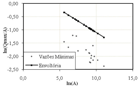
Figura 6 - Curva envoltória traçada para a região MAX II redefinida
