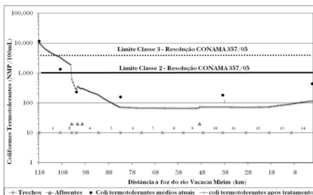
Figura 16 – Simulação dos coliformes termotolerantes para coleta/tratamento de esgotos de 50%
