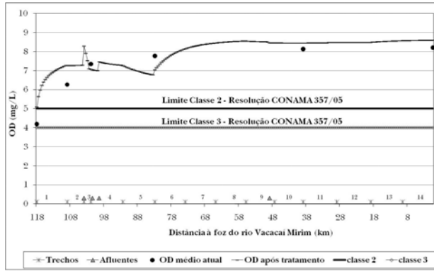
Figura 14 – Simulação do OD para coleta/tratamento de esgotos de 50%
