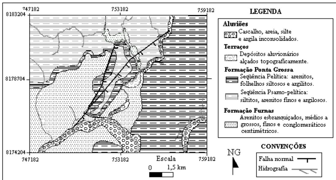
Figura 2 - Mapa geológico da região de Rondonópolis (Cutrim, 1999).
