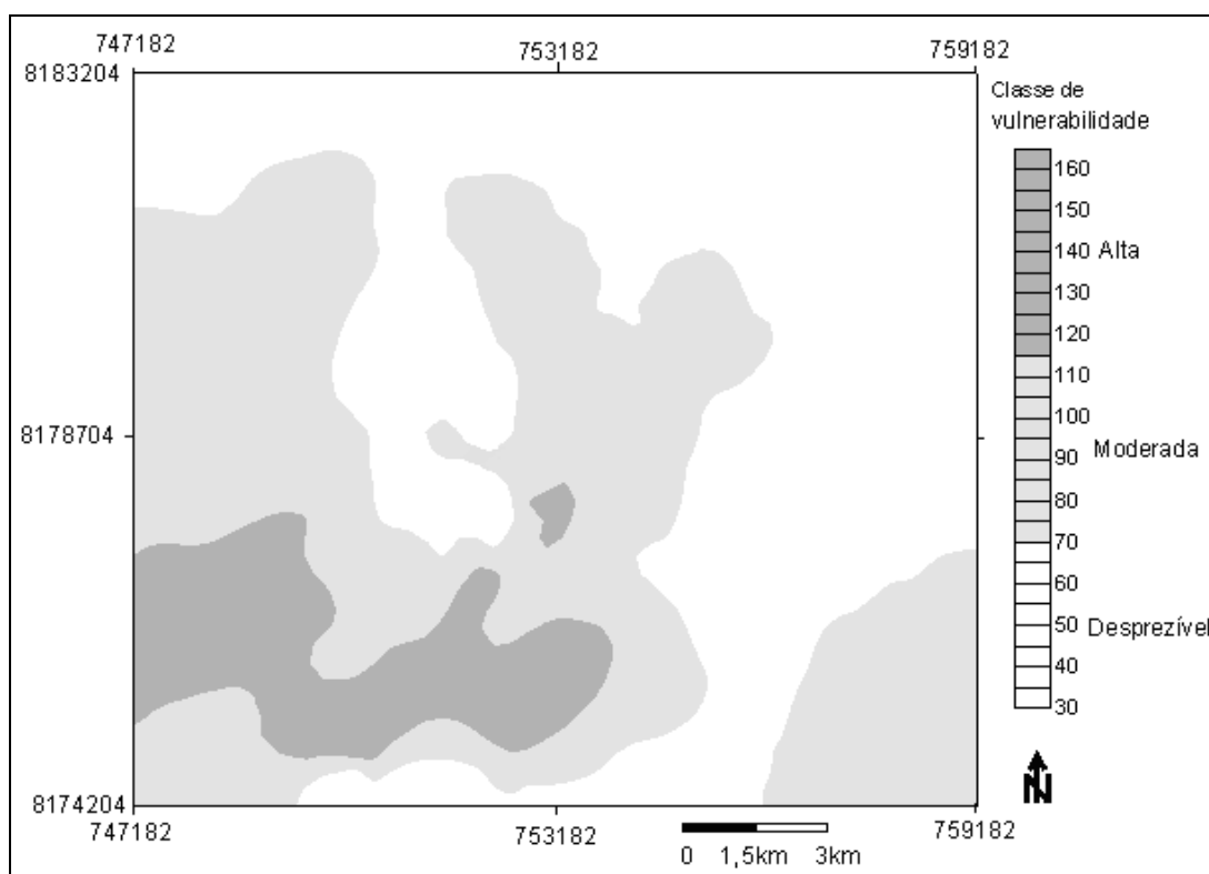
Figura 10 - Mapa de vulnerabilidade DRASTIC/modificado do Aquífero Furnas na cidade de Rondonópolis – MT.
