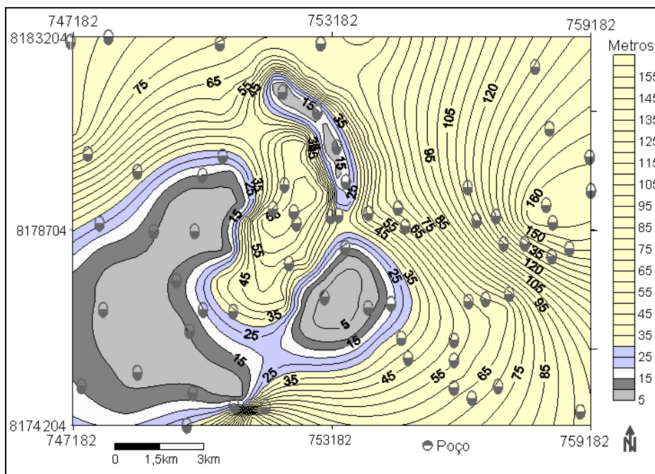
Figura 5 - Mapa potenciométrico do Aquífero Furnas na região de Rondonópolis.
