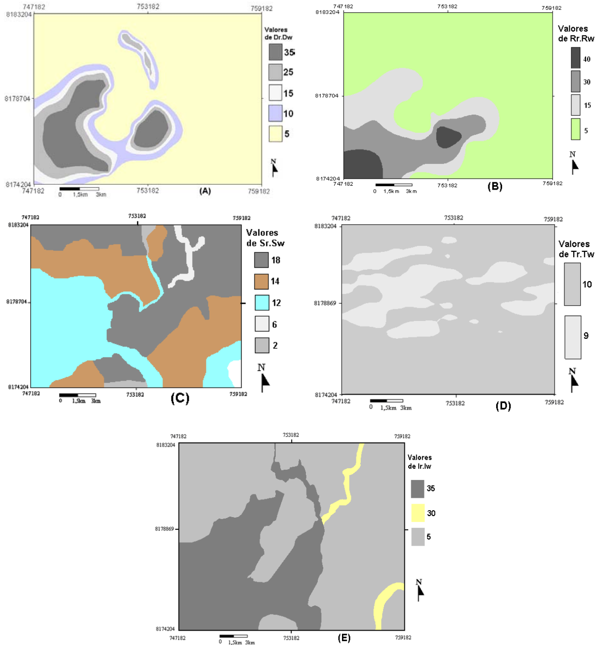
Figura 9 - Distribuição dos valores de Dr.Dw (A), Rr.Rw (B), Sr.Sw (C), Tr.Tw (D) e Ir.Iw (E) na área.
