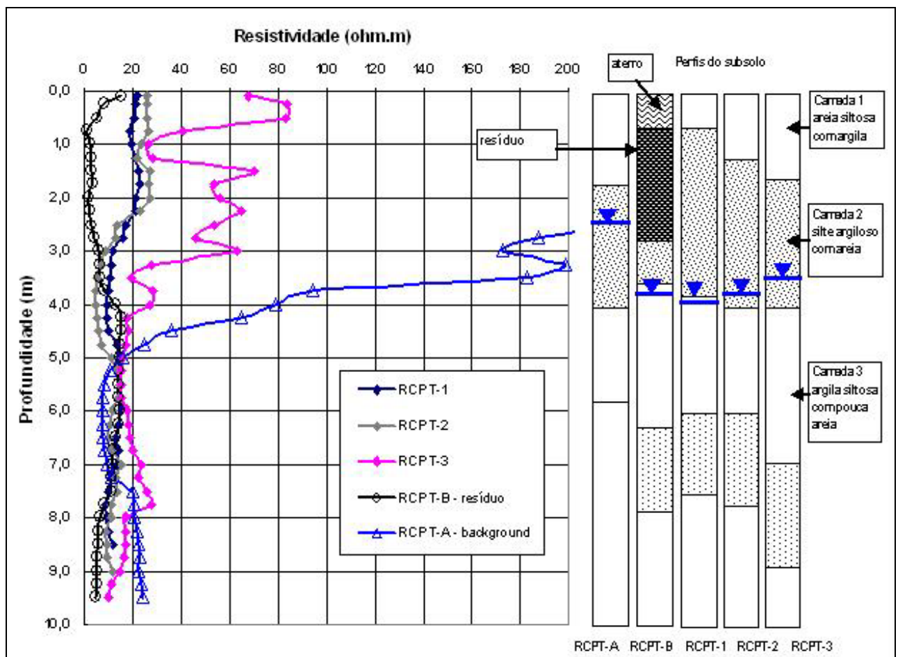
Figura 4 - Comparação dos ensaios de cone resistivo RCPT-1, RCPT-2, RCPT-3 e RCPT-B ( resíduo ) com o ensaio RCPT-A ( background ).
