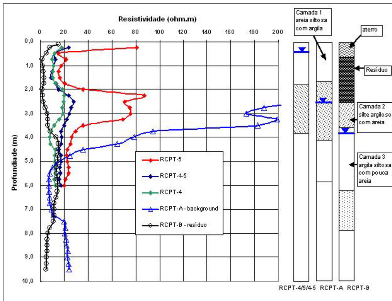
Figura 5 - Comparação dos ensaios de cone resistivo RCPT-4, RCPT-4-5, RCPT-5 e RCPT-B (resíduo) com o ensaio RCPT-A (background).
