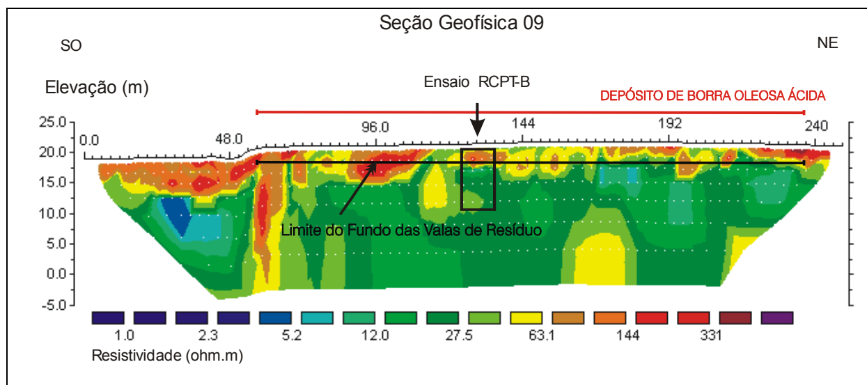
Figura 6 - Posição do ensaio RCPT-B sobre a seção geofísica 09.
