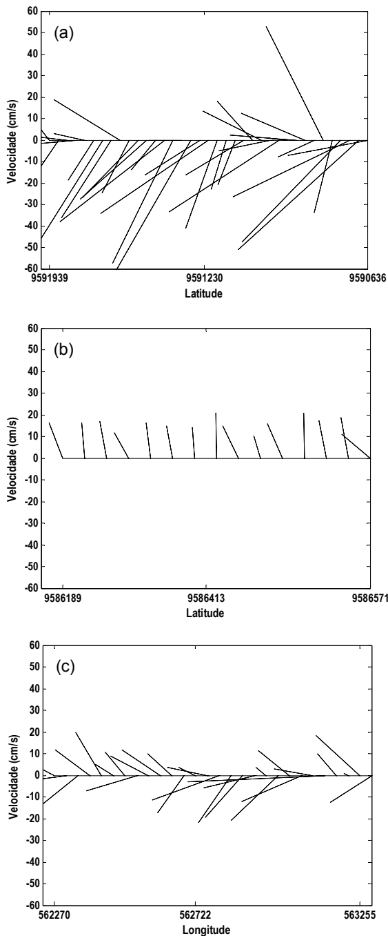
Figura 5 - Direção e intensidade das correntes em junho de 2008 no setor da costa Leste de Fortaleza: a) Perfil de ADP – P04; b) Perfil de ADP – P05; c) Perfil de ADP – P06.
